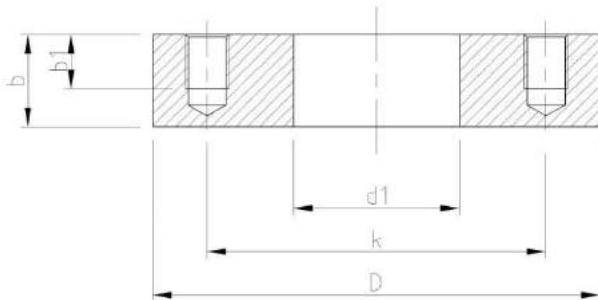
Schottflansch mit einseitigem Gewinde
