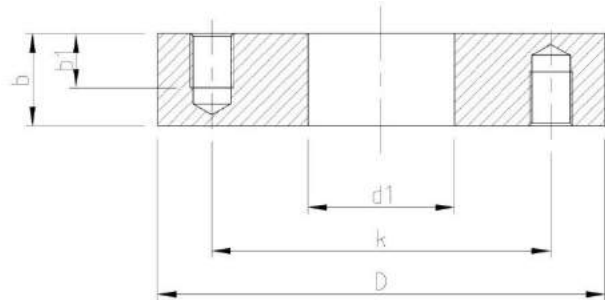
Schottflansch mit beidseitigem Gewinde
